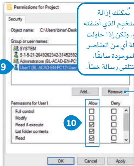
شكل 2.4: تعديل أذونات الملفات والمجلدات مُستخدم معيّن
