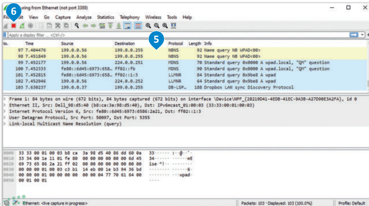
شكل 2.9: مراقبة الشبكة باستخدام واير شارك
