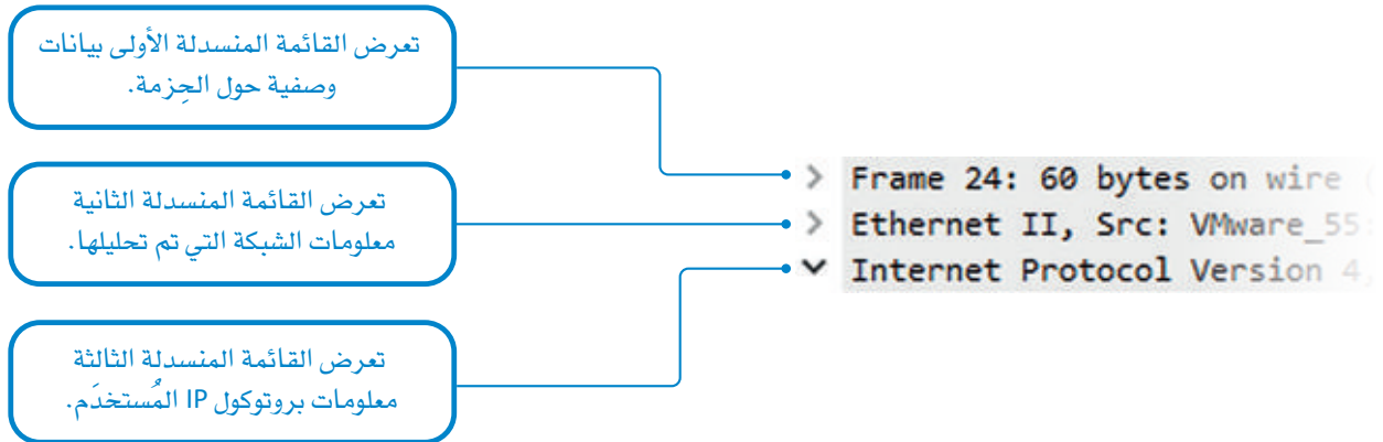
شكل 2.11: لوحة تفاصيل الحزمة
