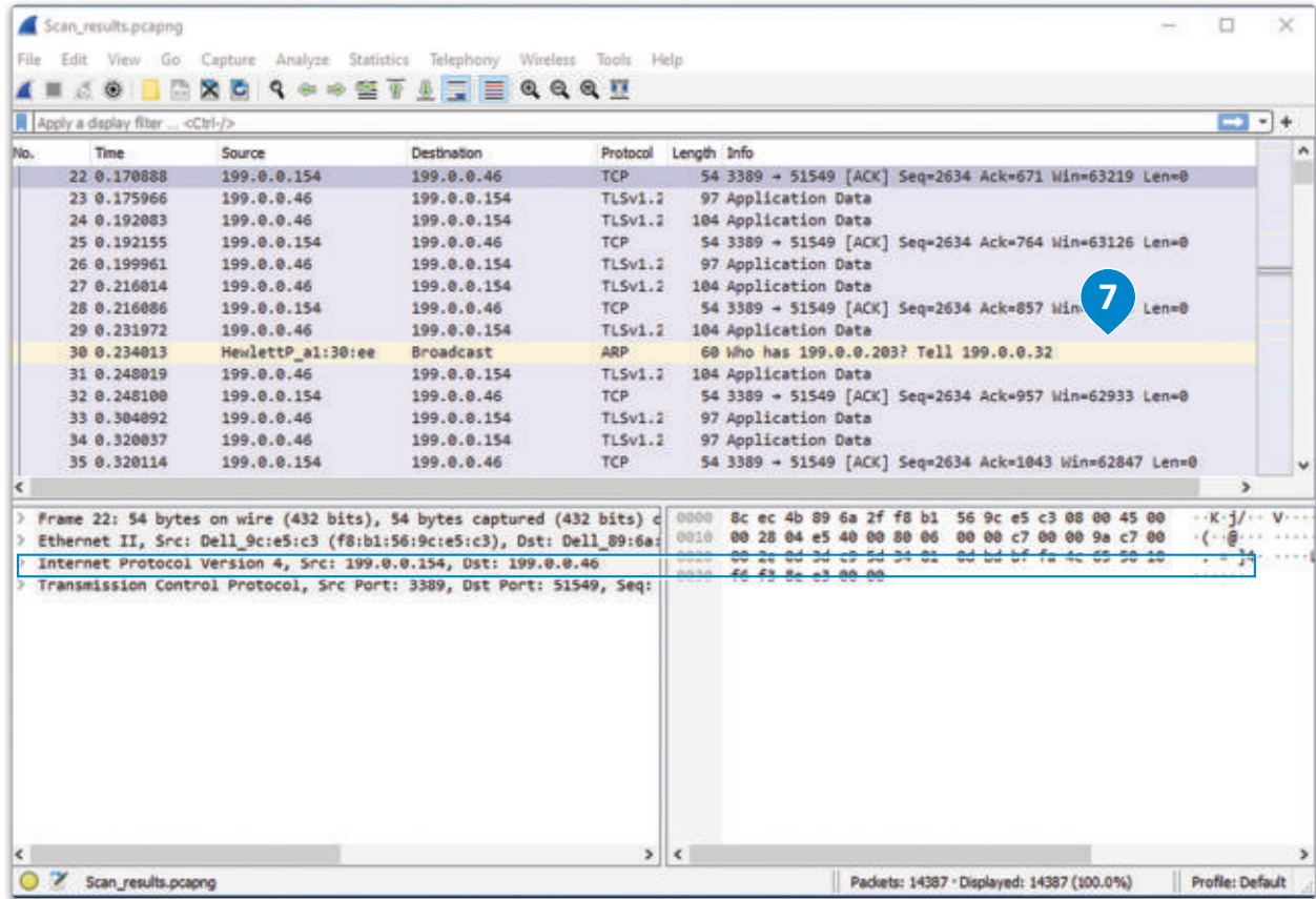
شكل 2.16: كشف طلبات بروتوكول اقتران العناوين (ARP)
