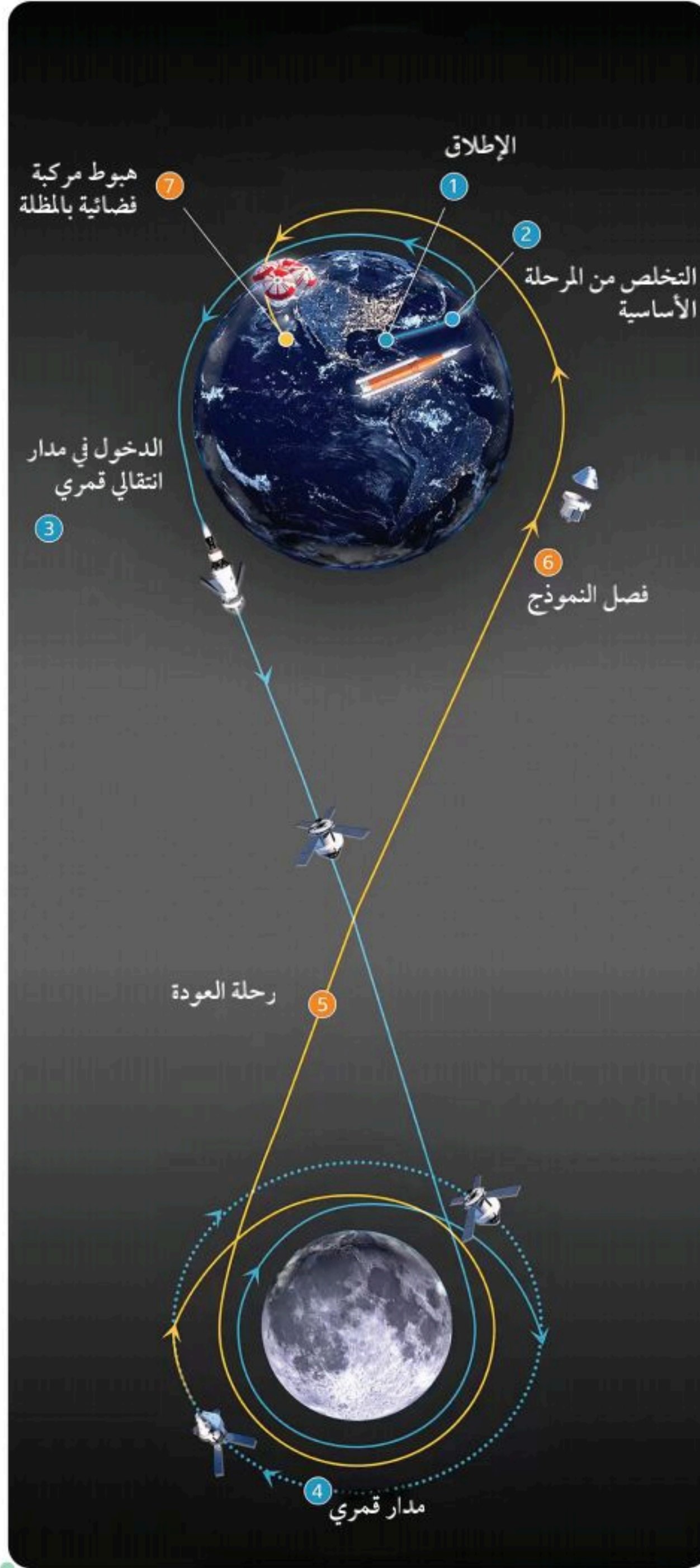
الشكل 9-2 رحلة مشروع أرتيمس للقمر.
