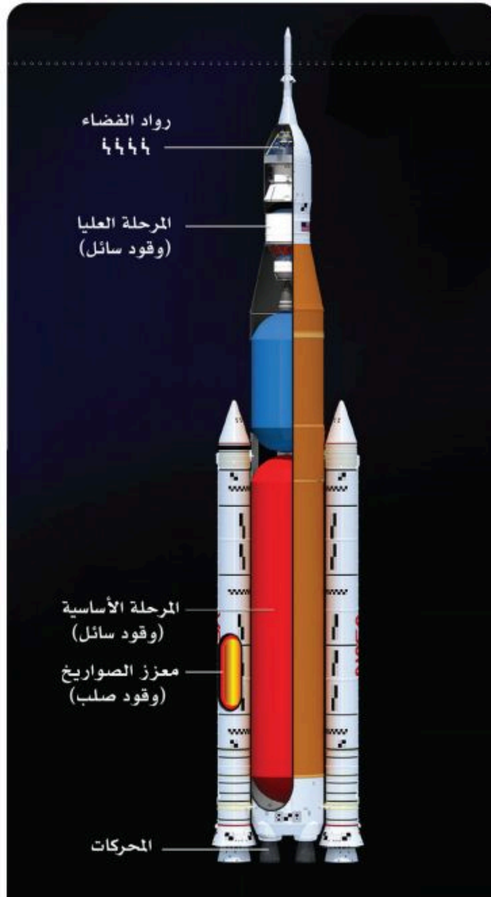
الشكل 19-2 تركيب صاروخ الإطلاق لمركبات الفضاء المأهولة.
