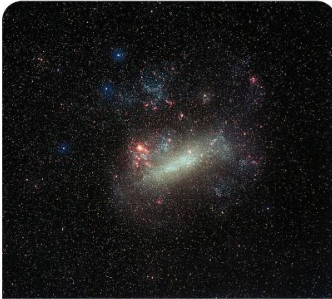
الشكل 1-18 مجرة سحابة ماجلان الكبرى غير المنتظمة.
