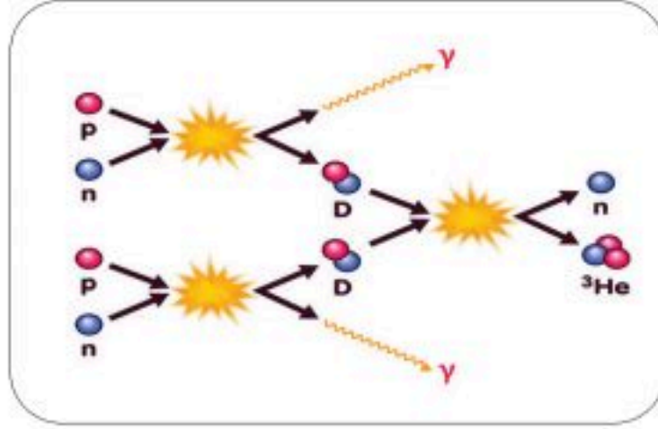
الشكل 1-3 اتحاد النيوترونات والبروتونات لتكوين ذرة الهيليوم.
