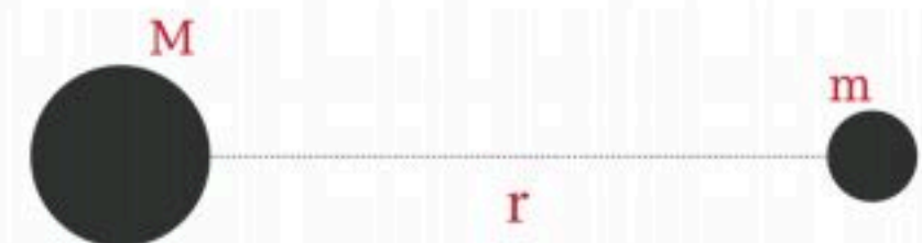
الشكل 7-2 قوة جذب كتلة الشمس على كتلة الأرض.
