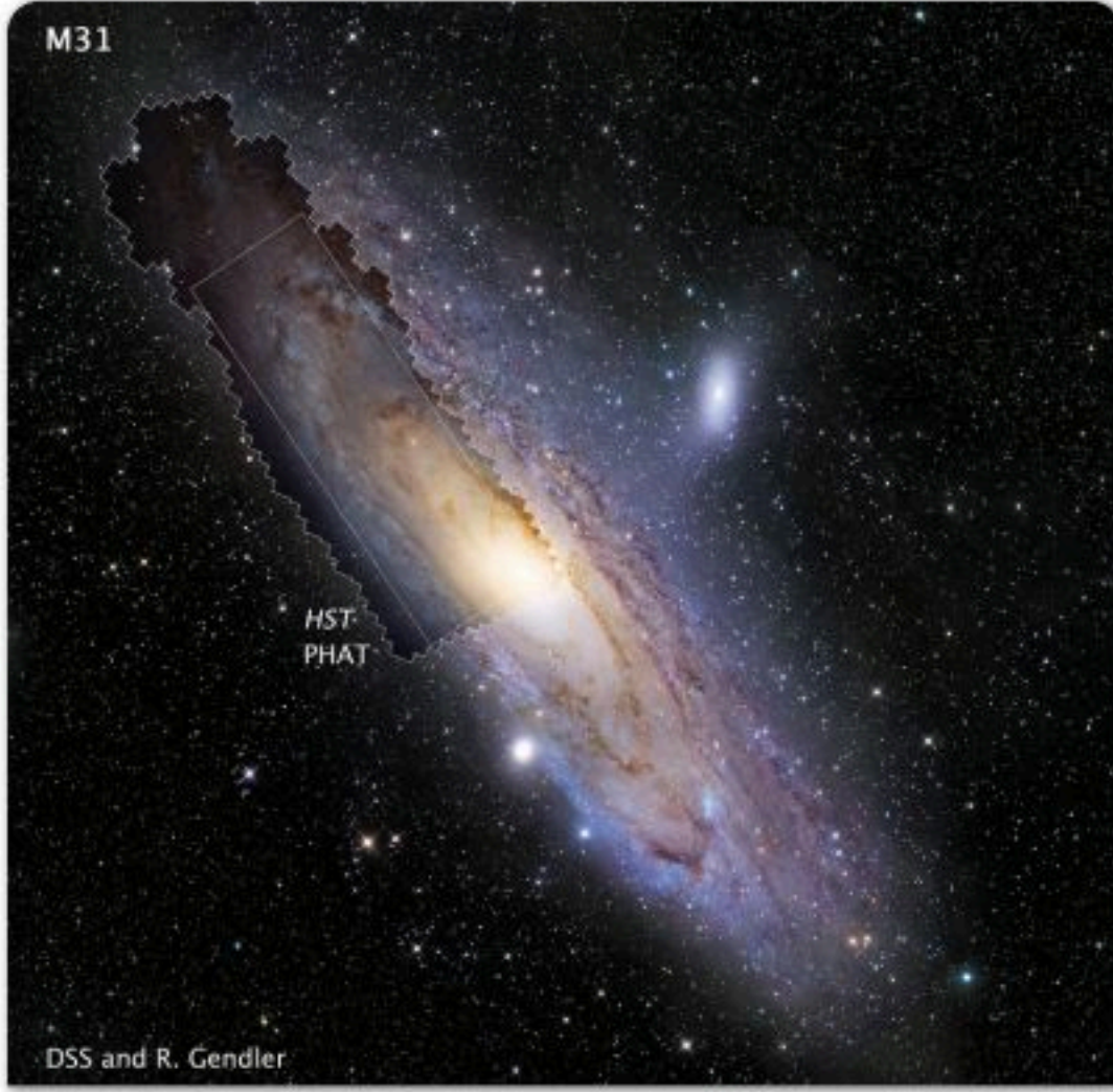
الشكل 1-16 مجرة المرأة المسلسلة إحدى المجرات الحلزونية.
