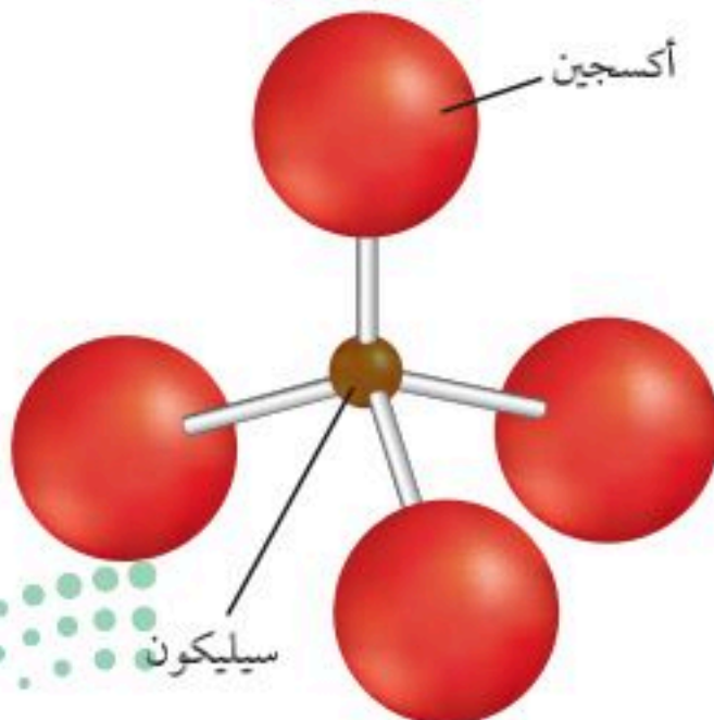
نموذج هرم رباعي الأوجه
