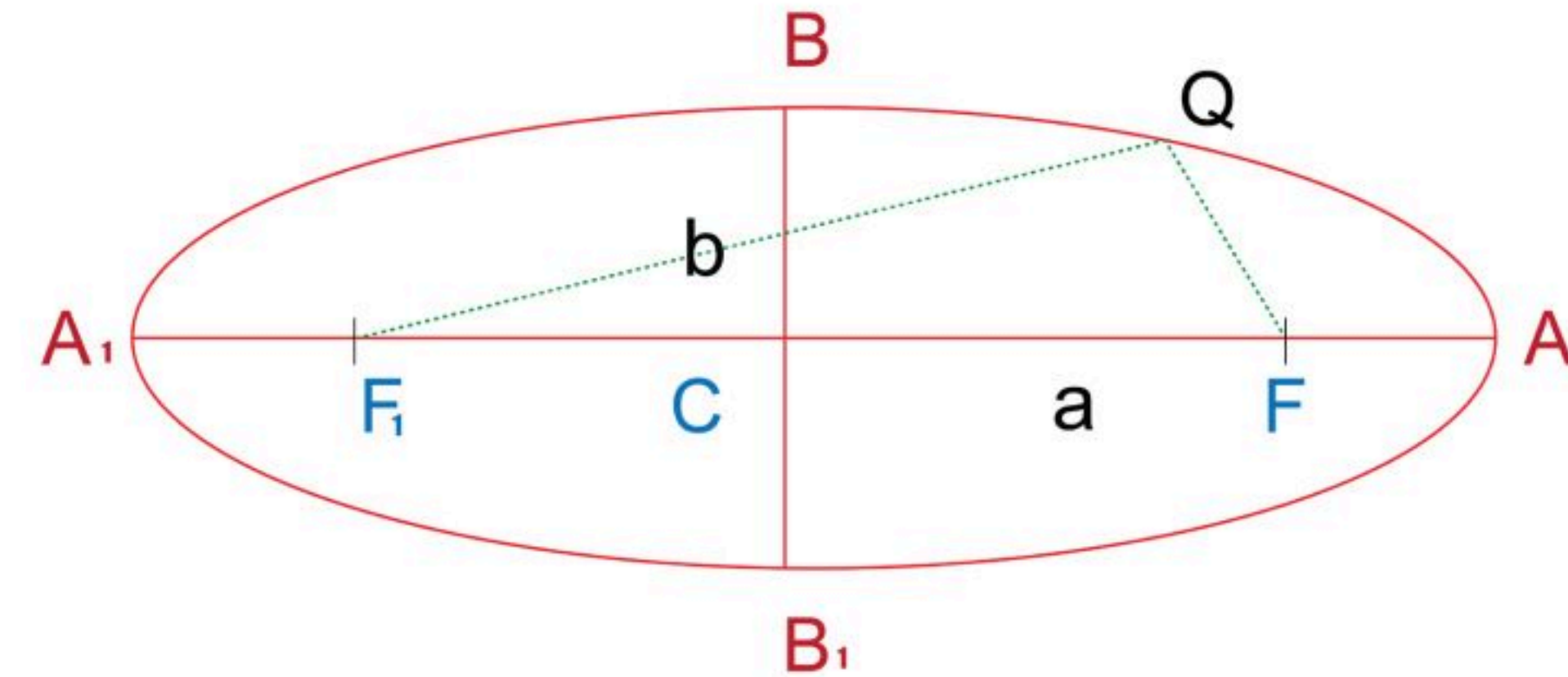
الشكل 2-3 خصائص القطع الناقص.
