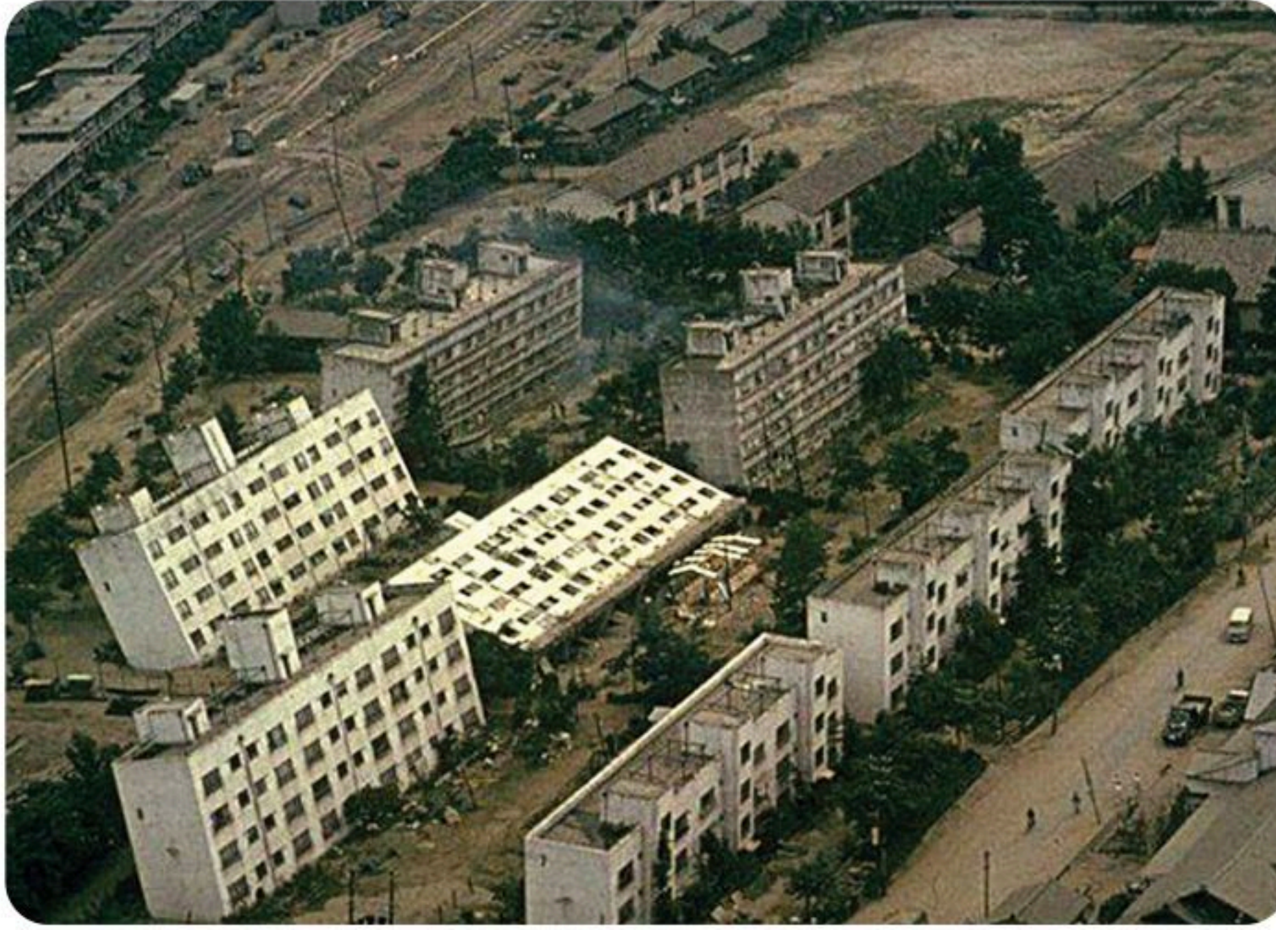
الشكل 35-6 يحدث تسييل في التربة الضعيفة التماسك عندما تنتشر اهتزازات زلزالية فيها، فتسلك سلوك الرمال المتحركة.
