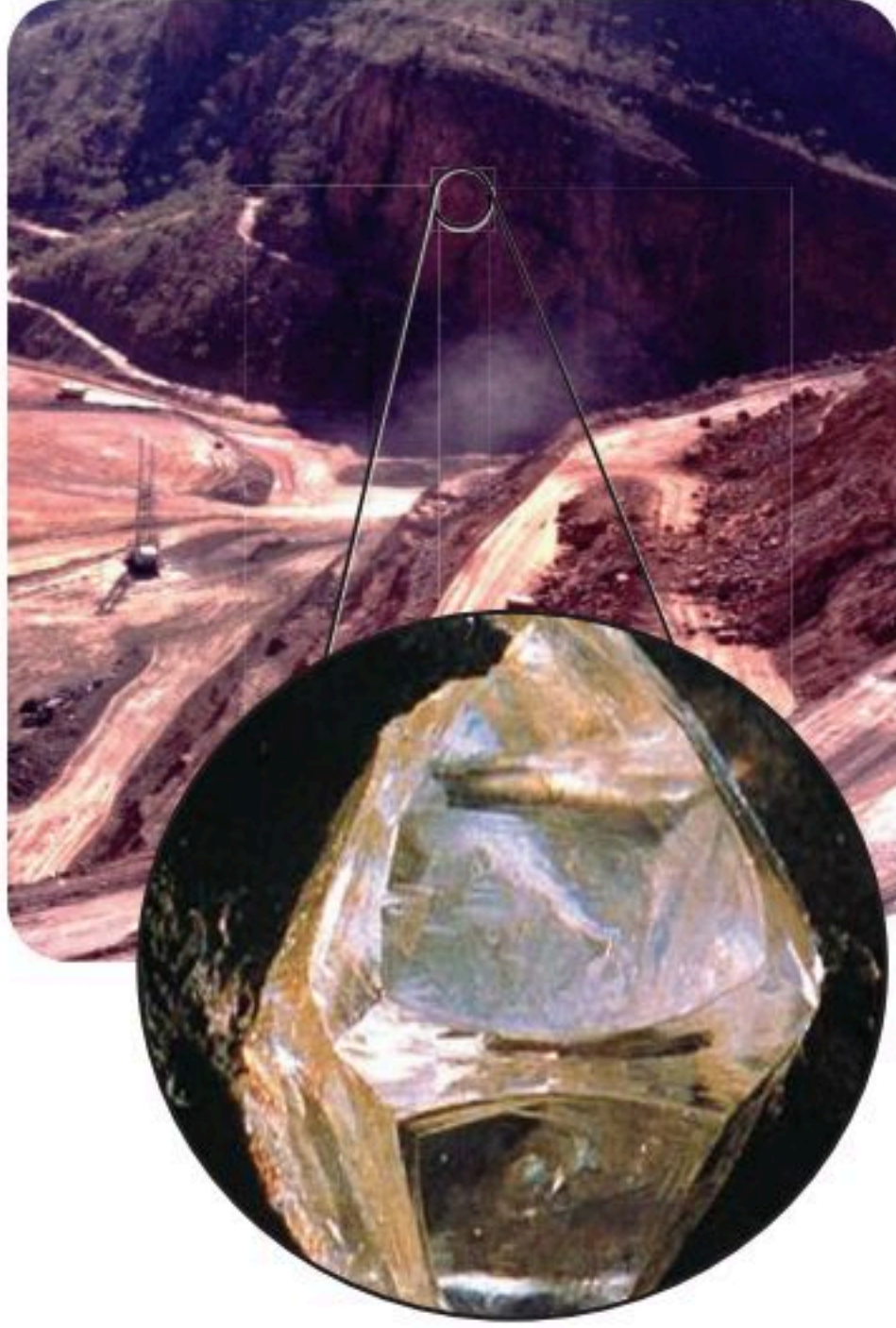
الشكل 14-4 يستخرج الألماس من الكمبرليت في منجم في جنوب إفريقيا.
