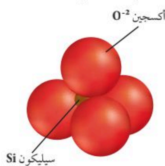
منظر مصمت لهرم سيليكات رباعي الأوجه
