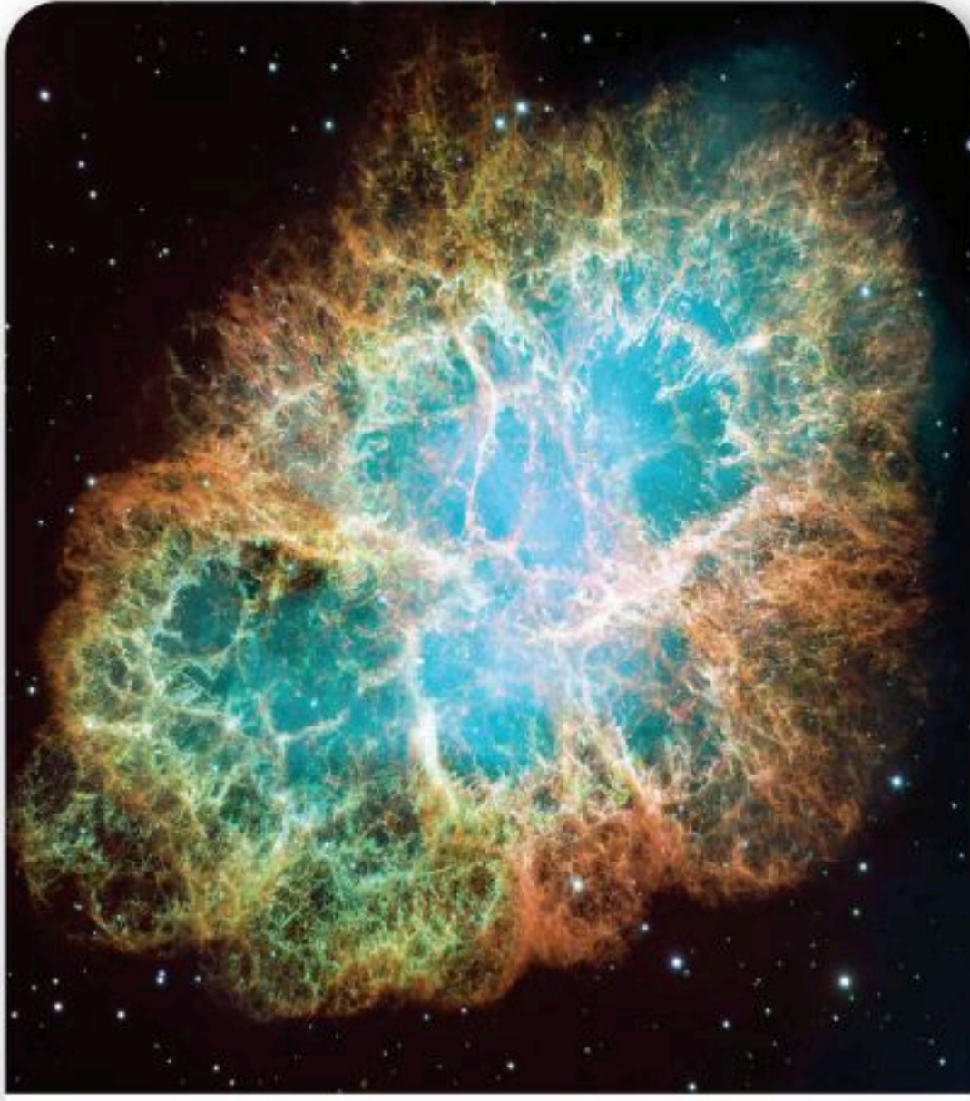
الشكل 1-14 سديم السرطان، وهو بقايا نجم ضخم من مجرتنا، تمت رؤية انفجاره في عام 1054.
