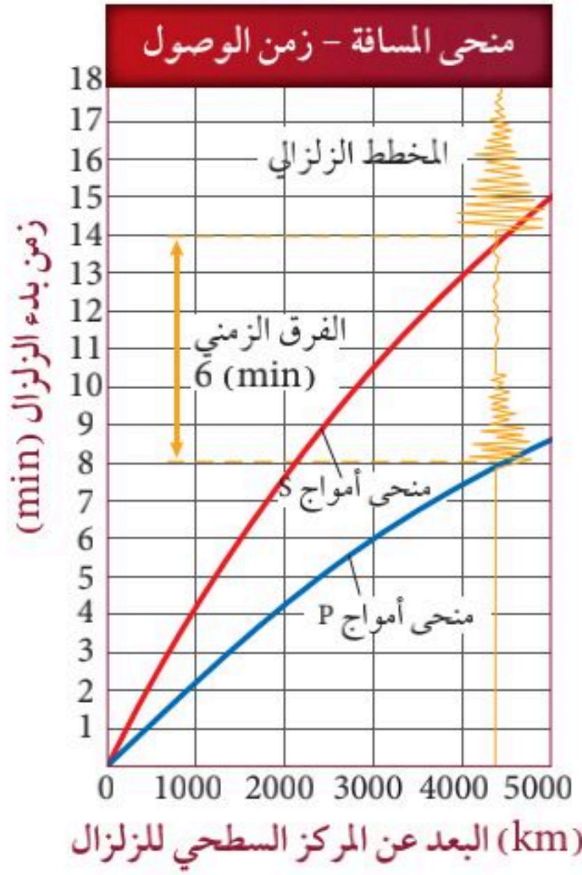
الشكل 29-6 يبين منحنى (المسافة- الزمن) الوصول هذا بيانات زلزالية لزلزال ما.
