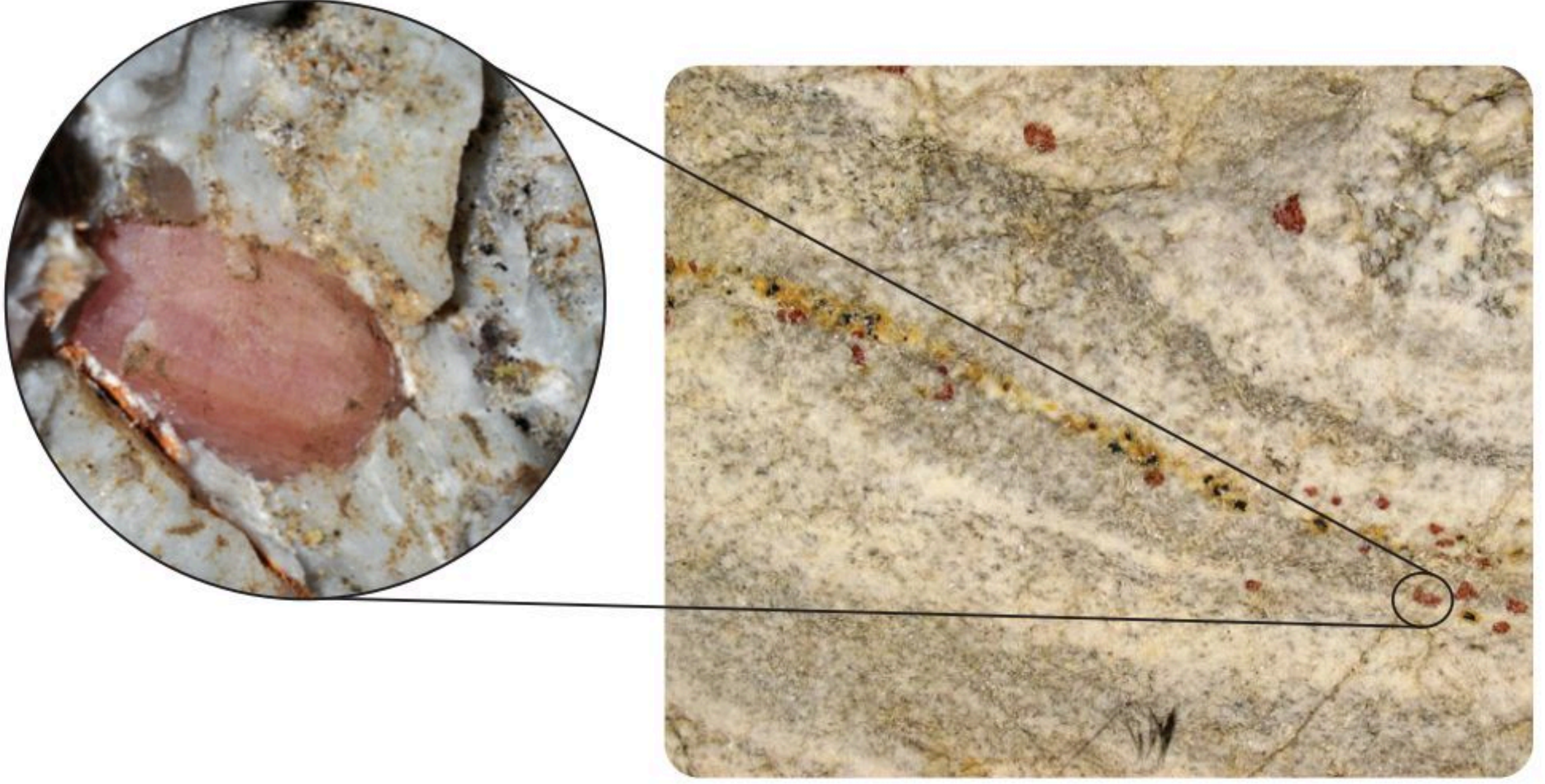
الشكل 13-4 عرق بيجماتيت يخترق صخور الجرانيت، وفيه بلورات جميلة.
