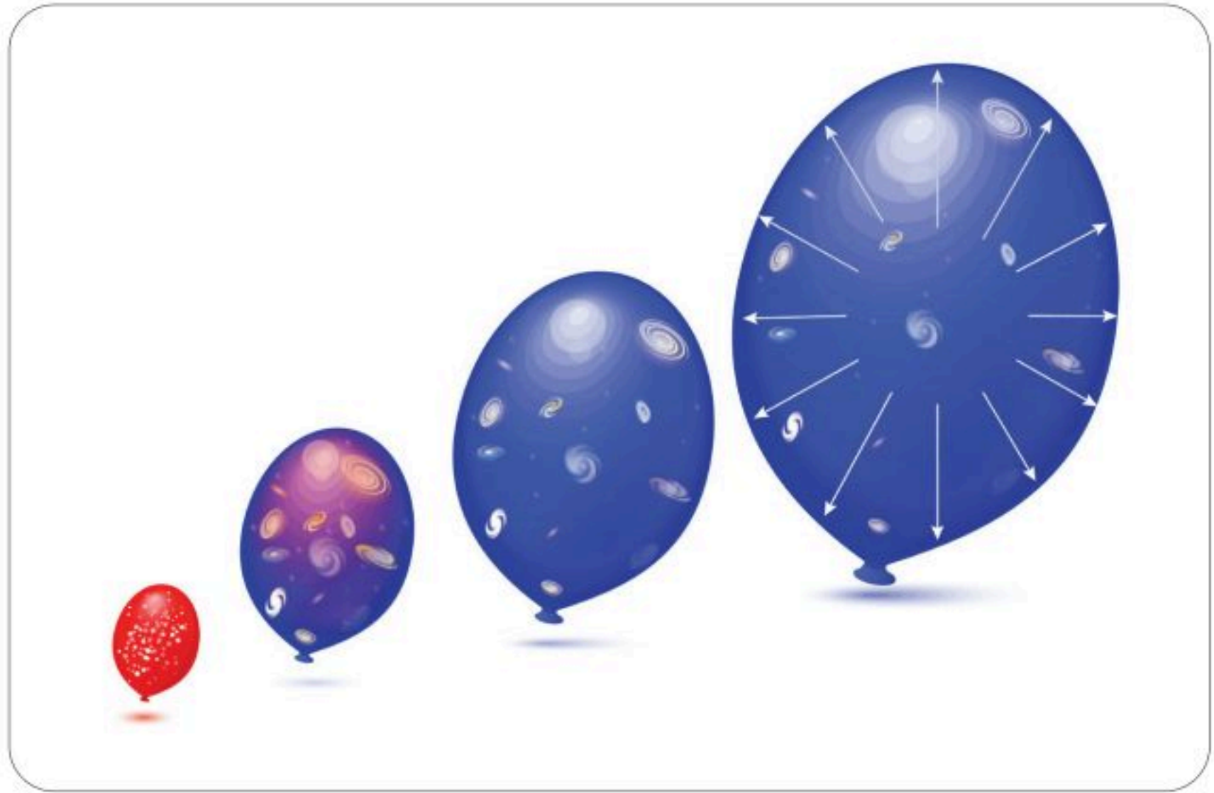
الشكل 1-7 يوضح تصور تمدد الكون.
