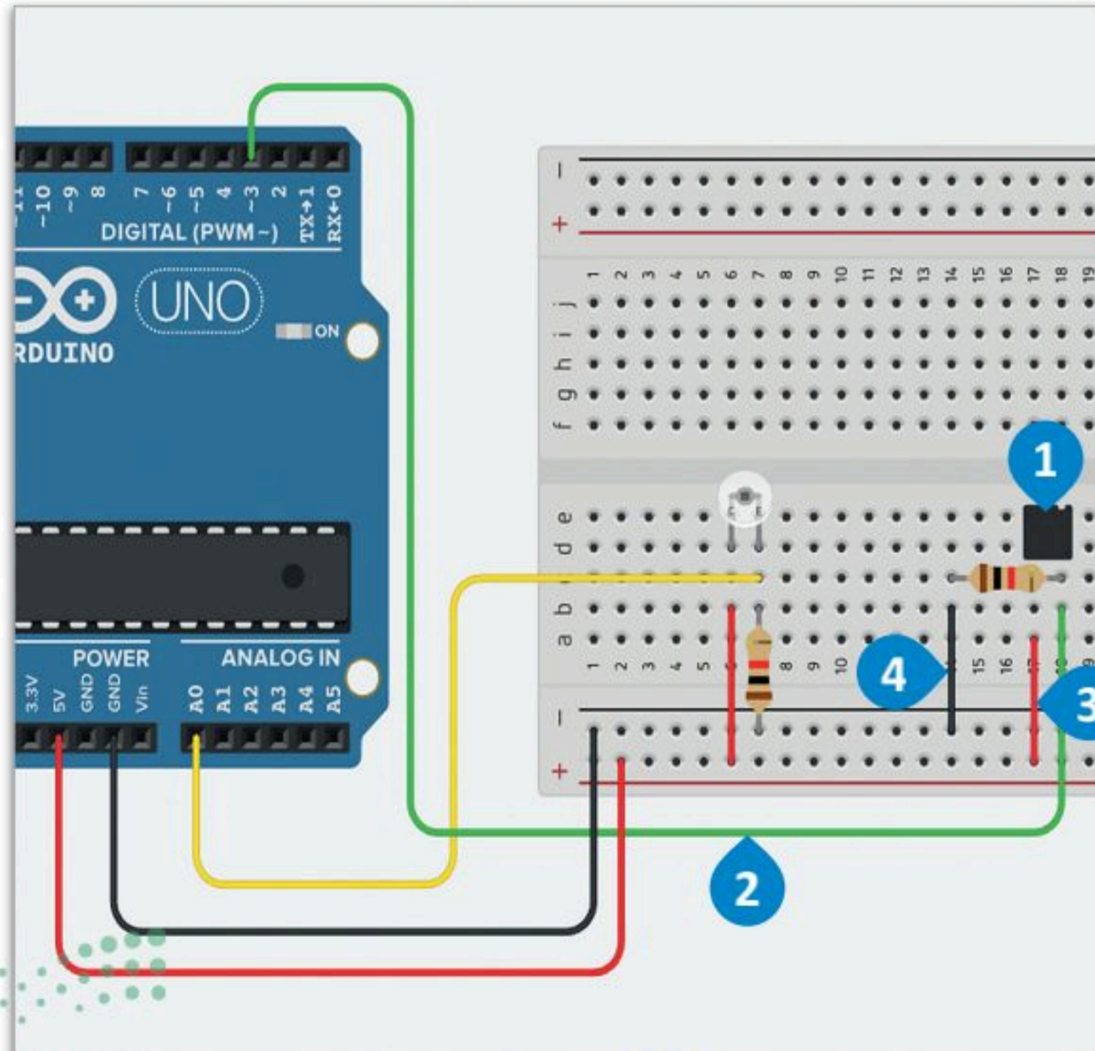
شكل 7.15: توصيل مُستشعر الإمالة
