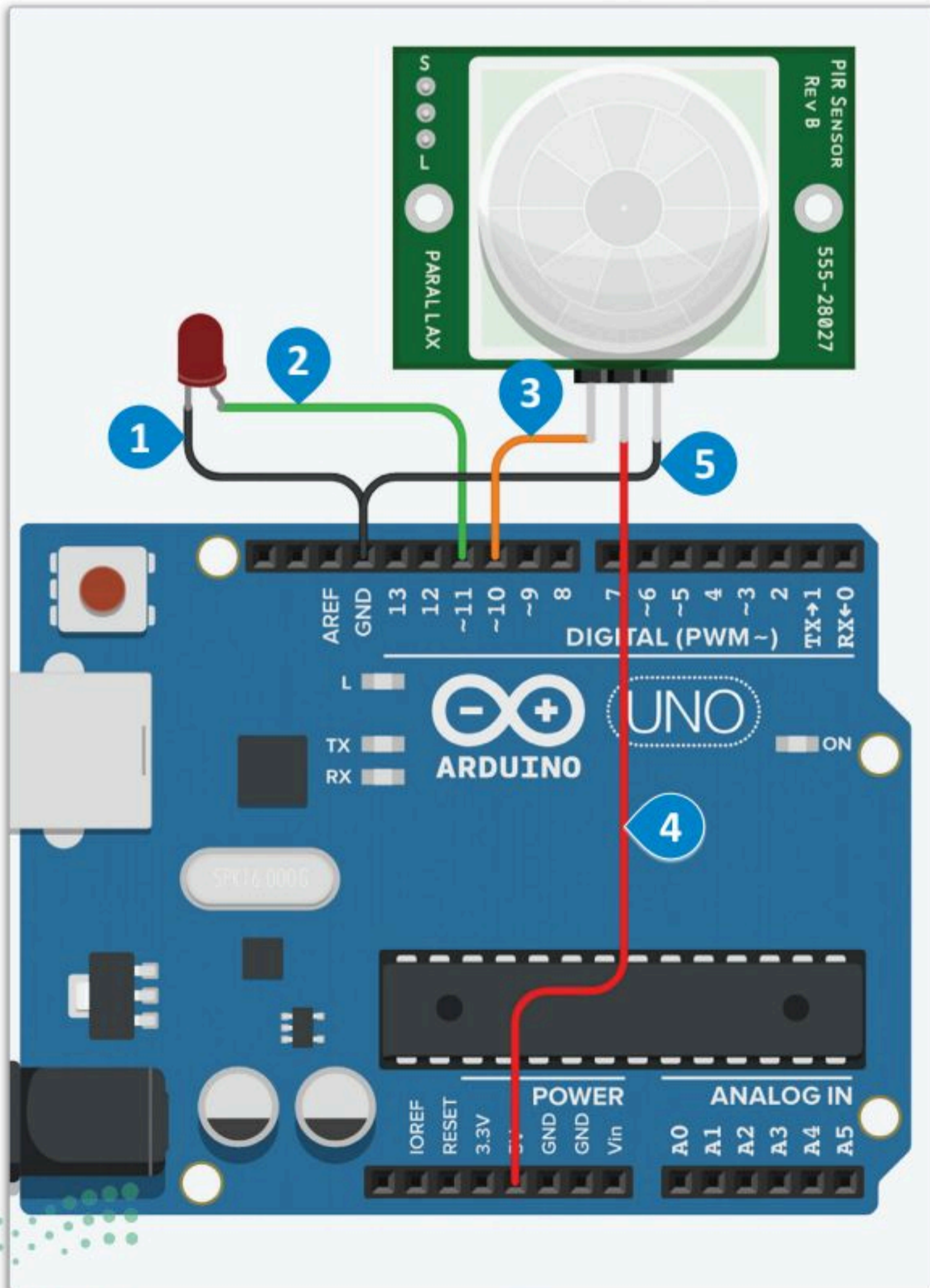
شكل 6.14: توصيل الدائرة
