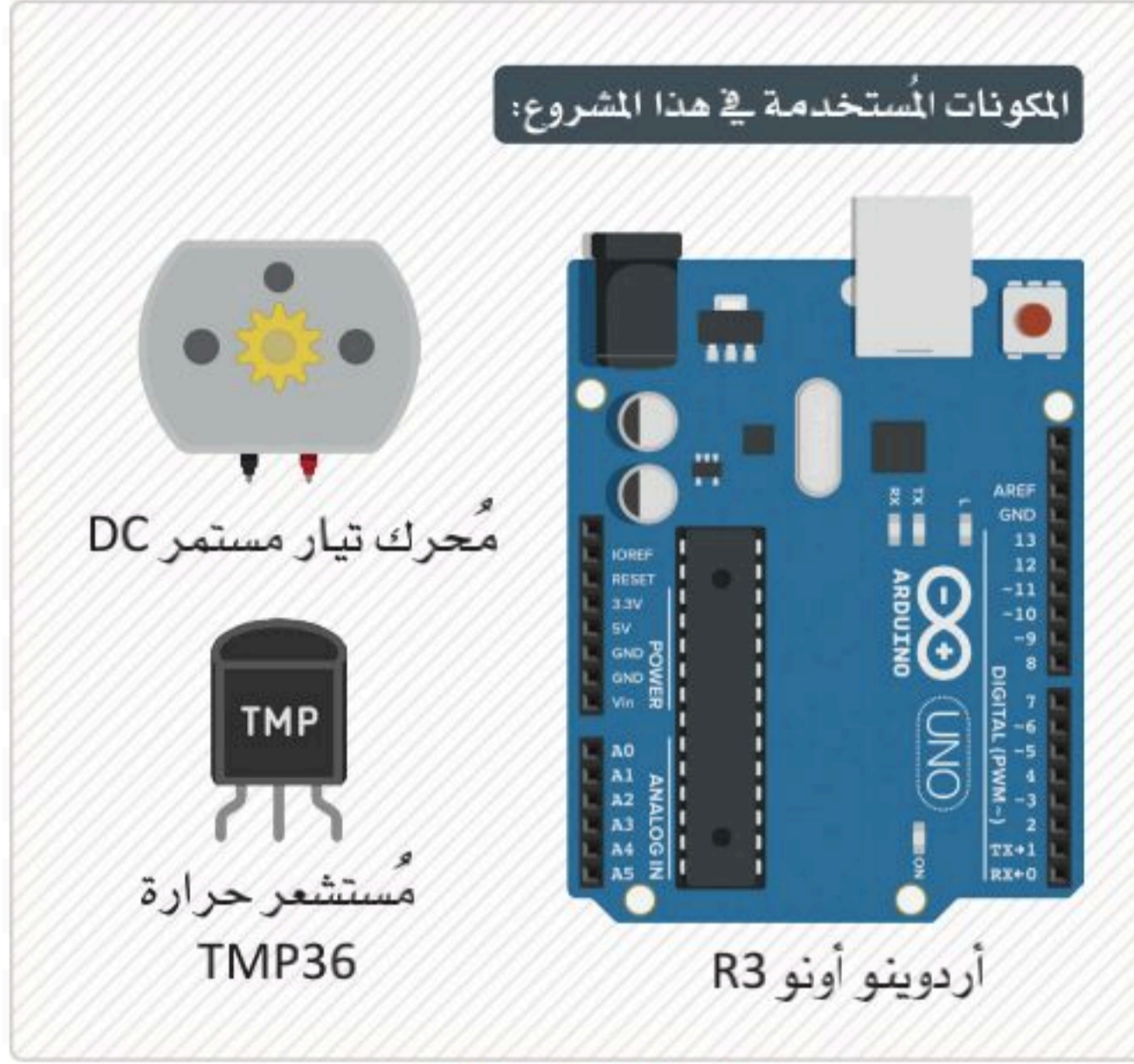
شكل 6.15: مكونات المشروع
