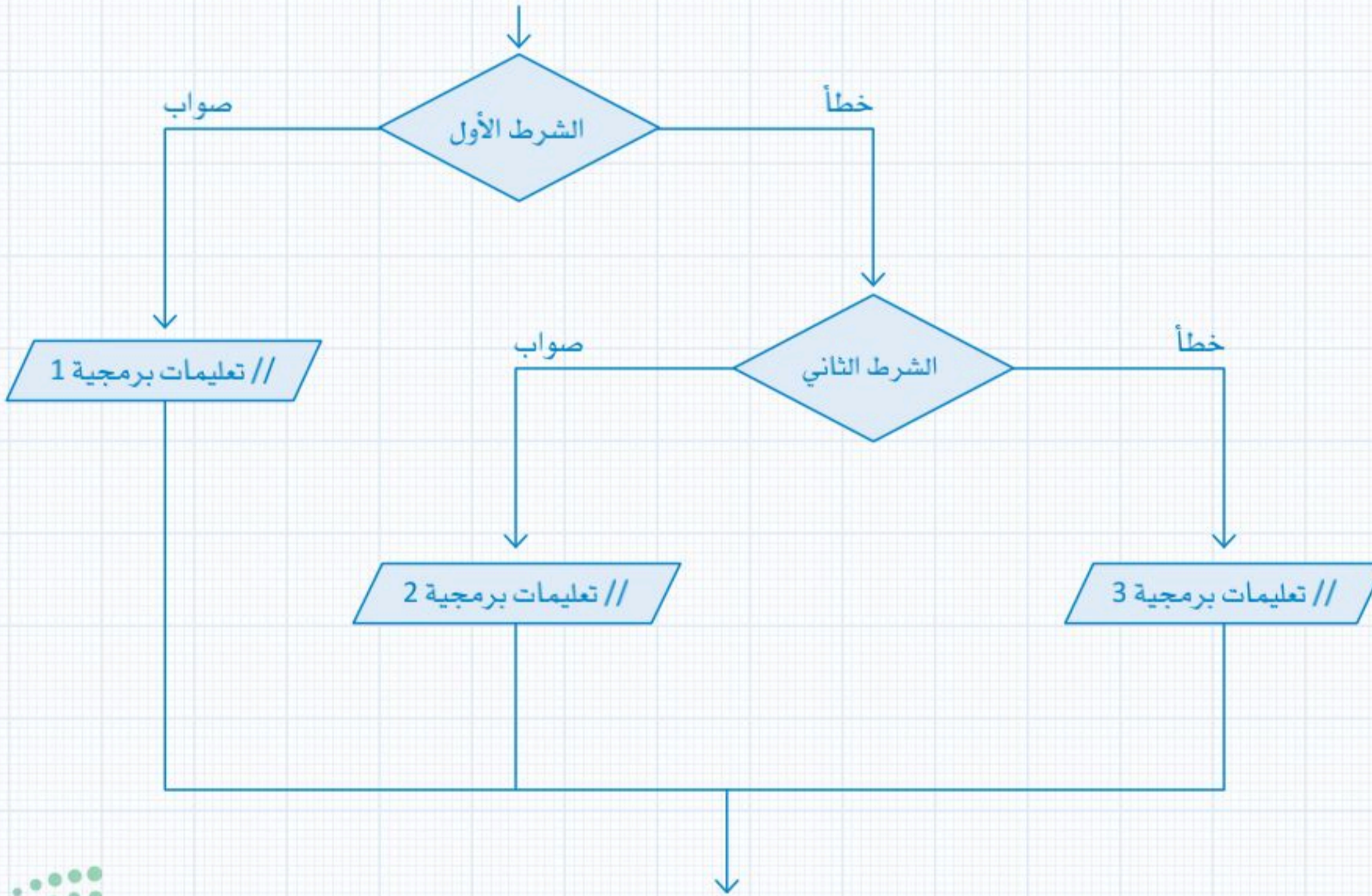
شكل 6.4: مخطط عبارة if .. else if .. else
