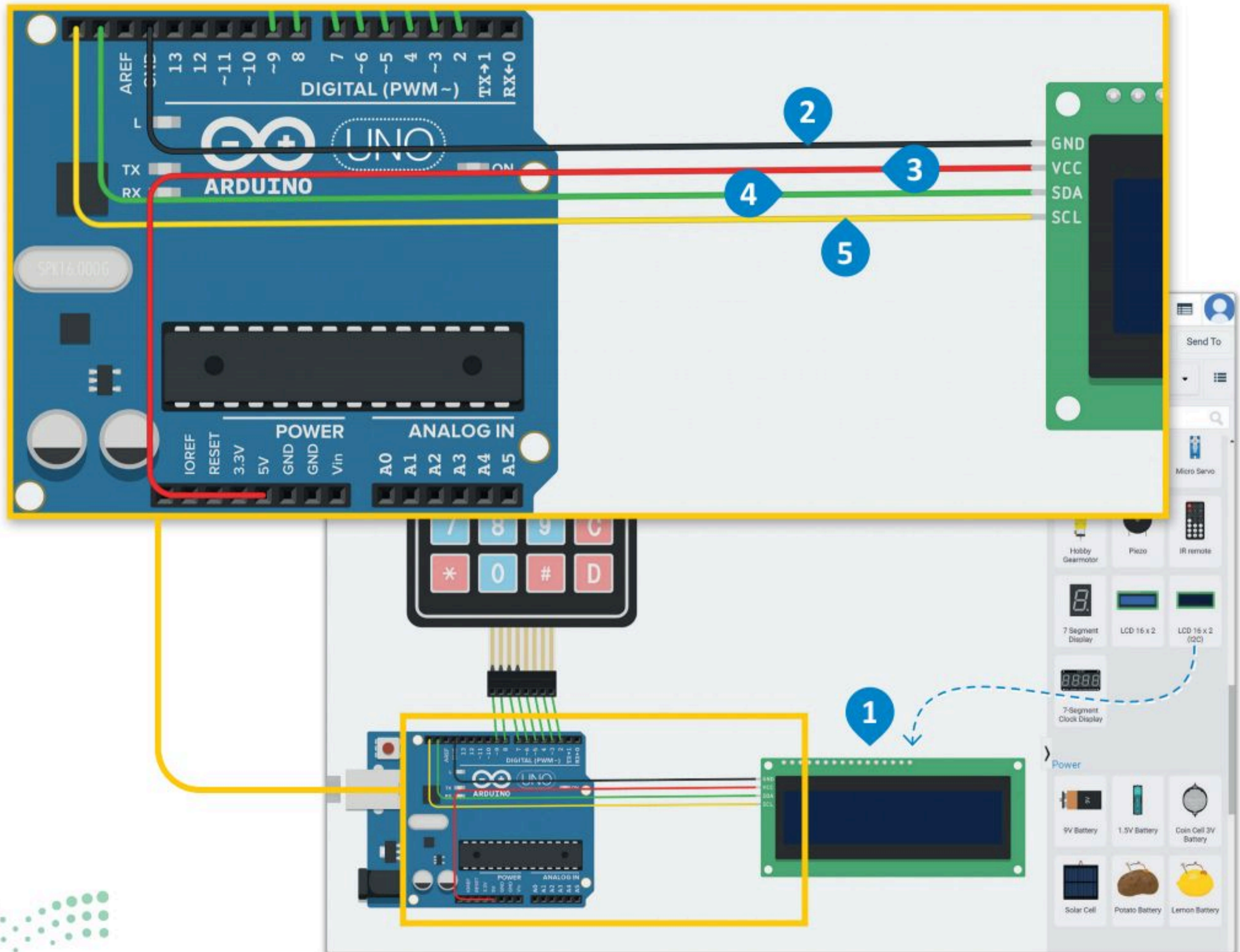
شكل 6.19: توصيل شاشة LCD
