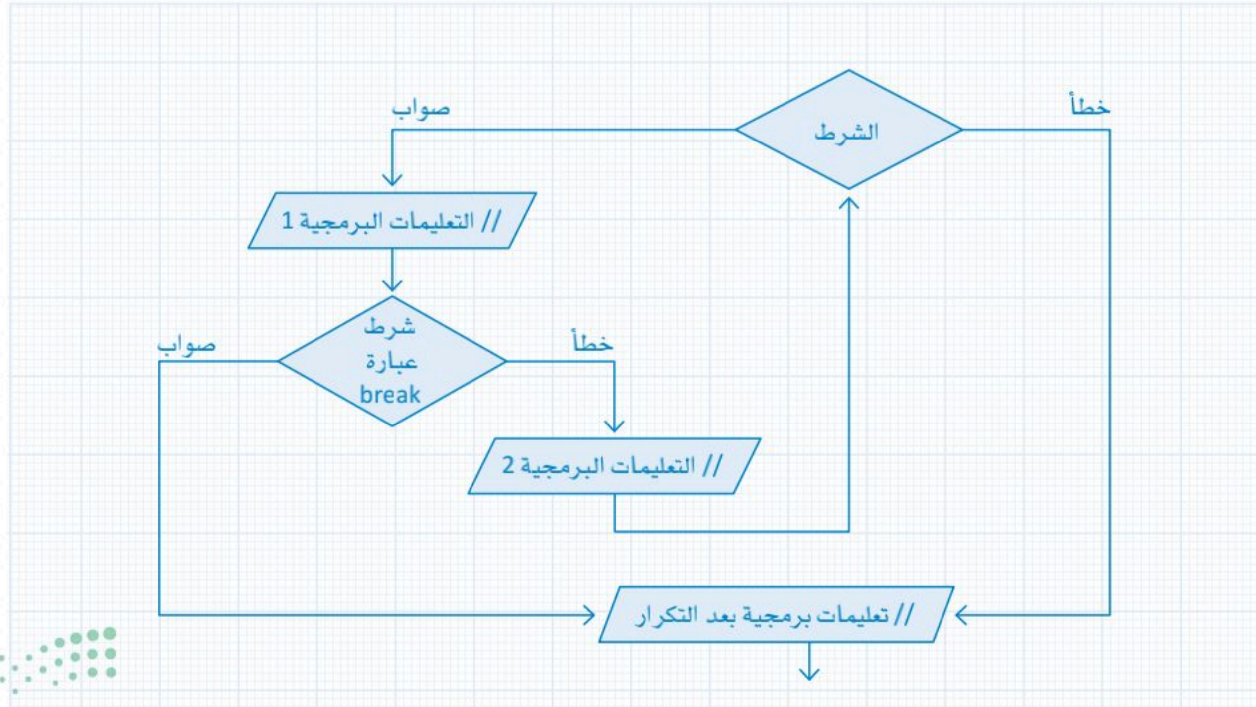
شكل 6.8: مخطط عبارة break
