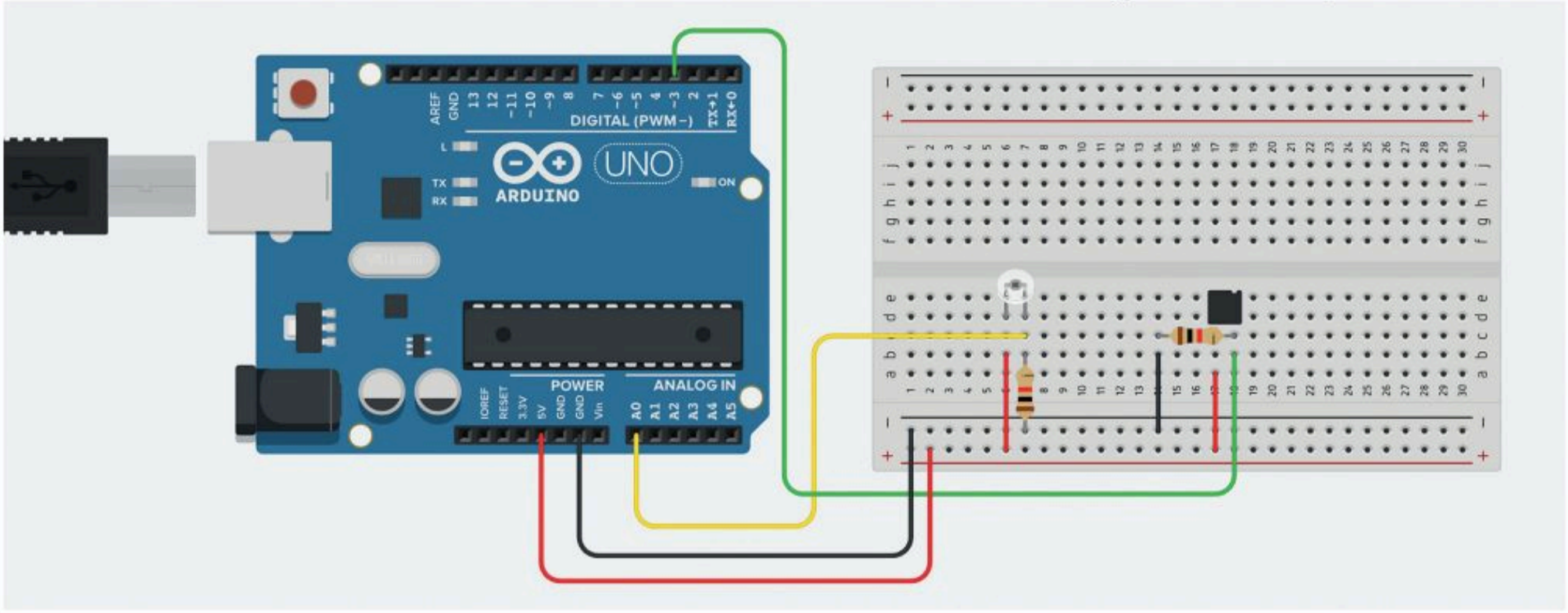
شكل 7.16: الدائرة بصورتها النهائية في تنكر كاد
