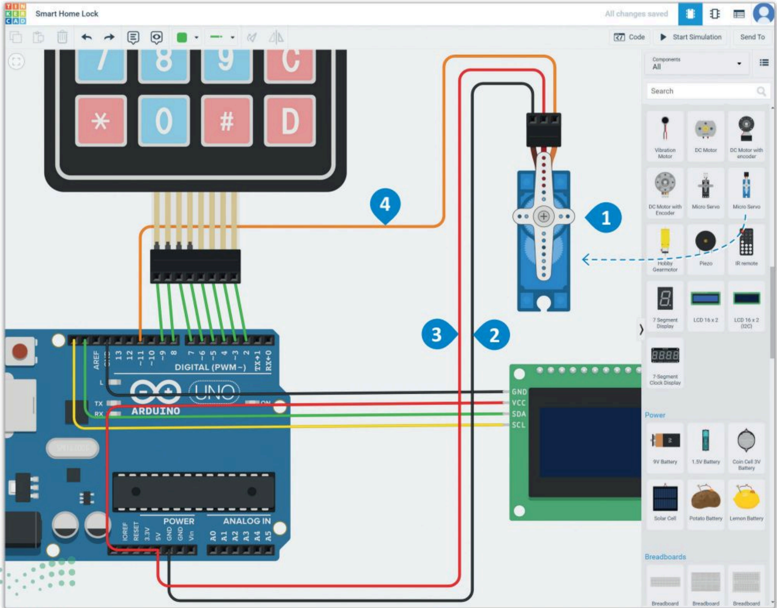
شكل 6.20: توصيل محرك السيرفو المصغر
