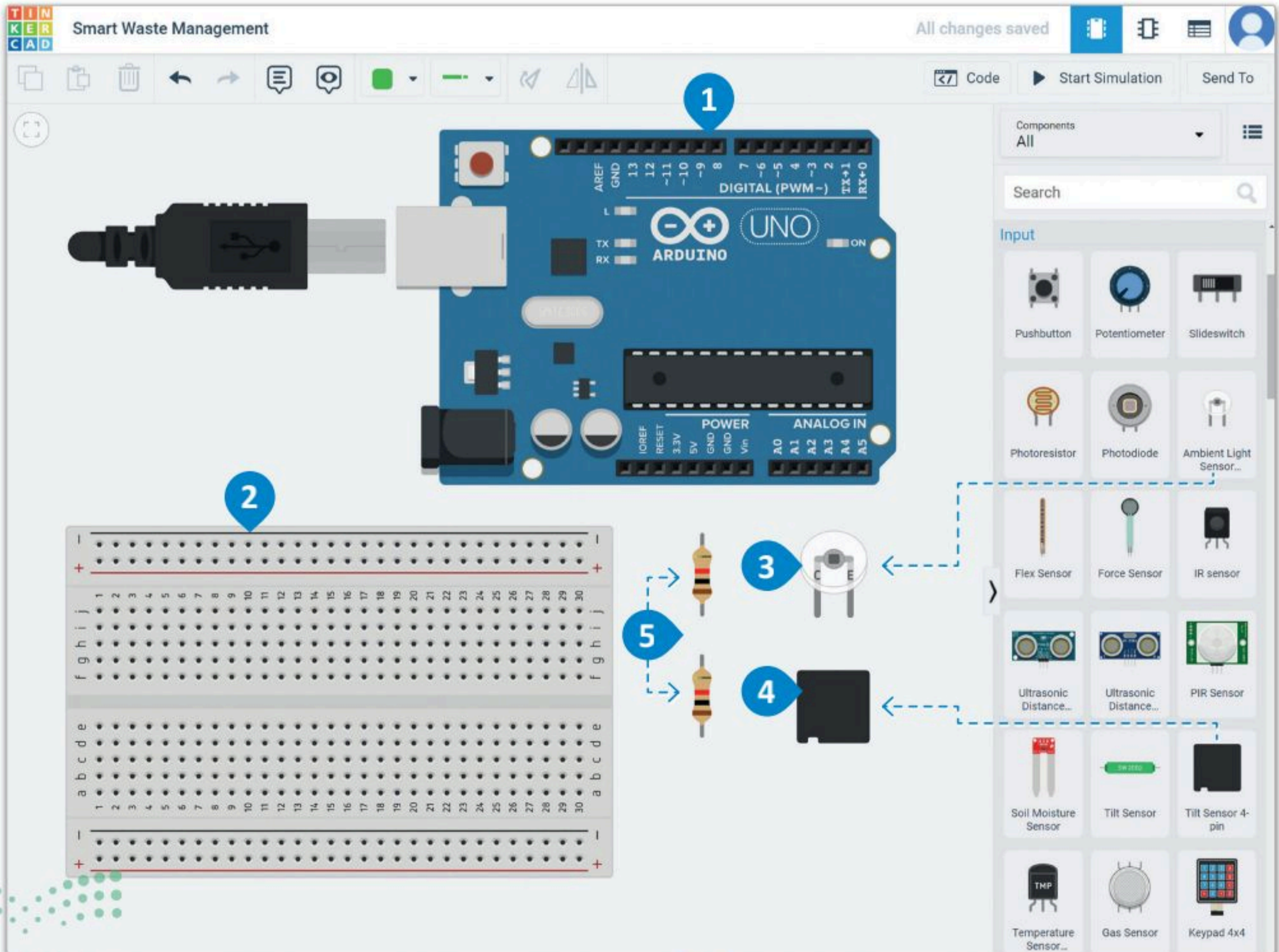
شكل 7.13: تثبيت مكونات الدائرة
