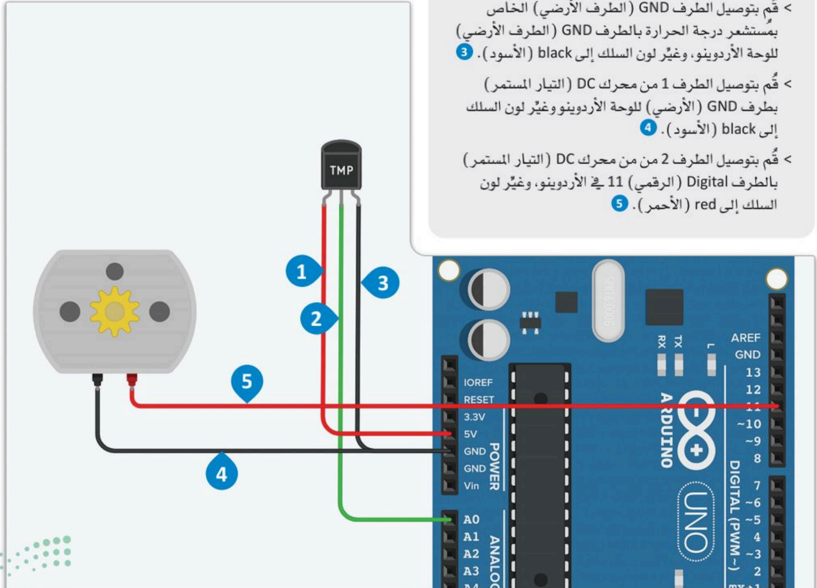
شكل 6.16: توصيل الدائرة
