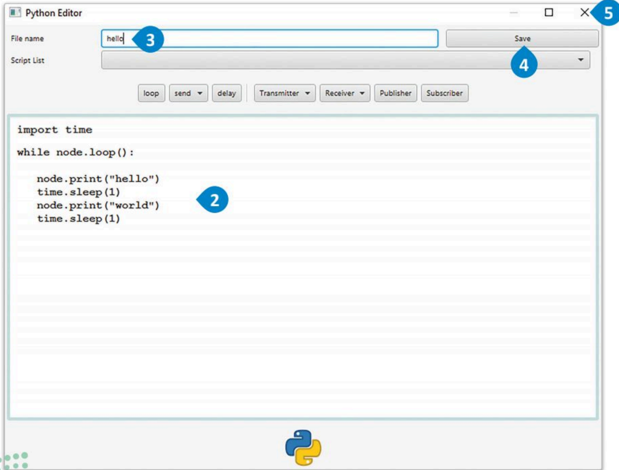
شكل 8.9: مُحرر البايثون
