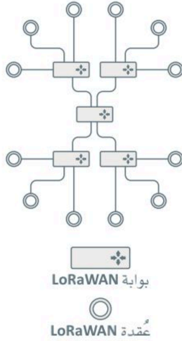
شكل 5.27: هيكلية LoRaWAN "نجمة النجوم"
