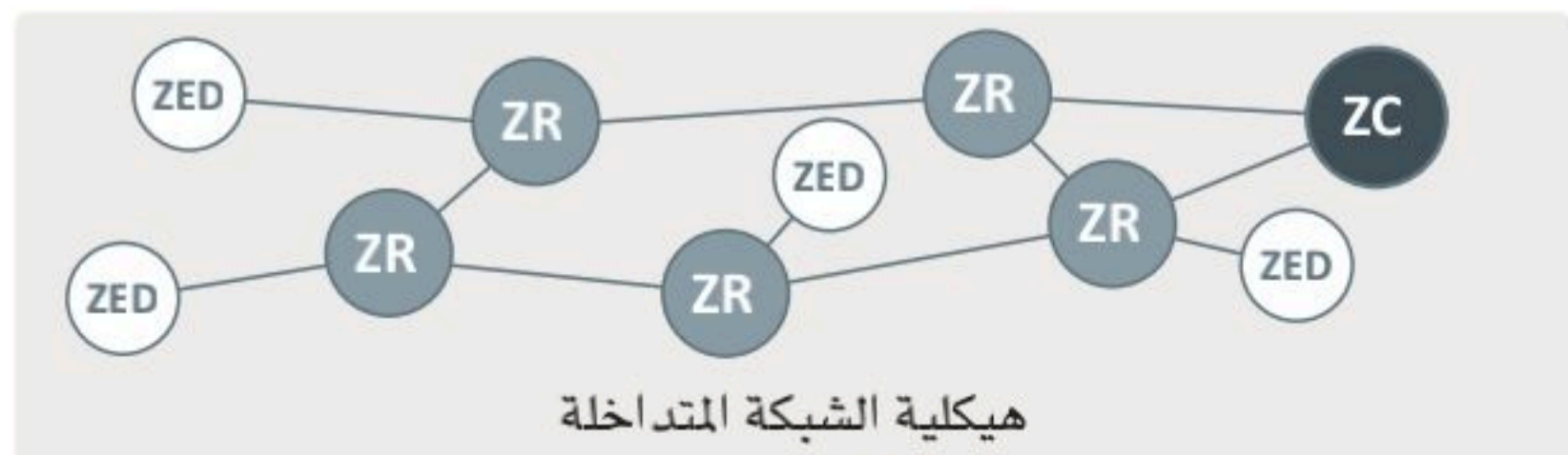
شكل 5.23: هيكليات زيجبي
