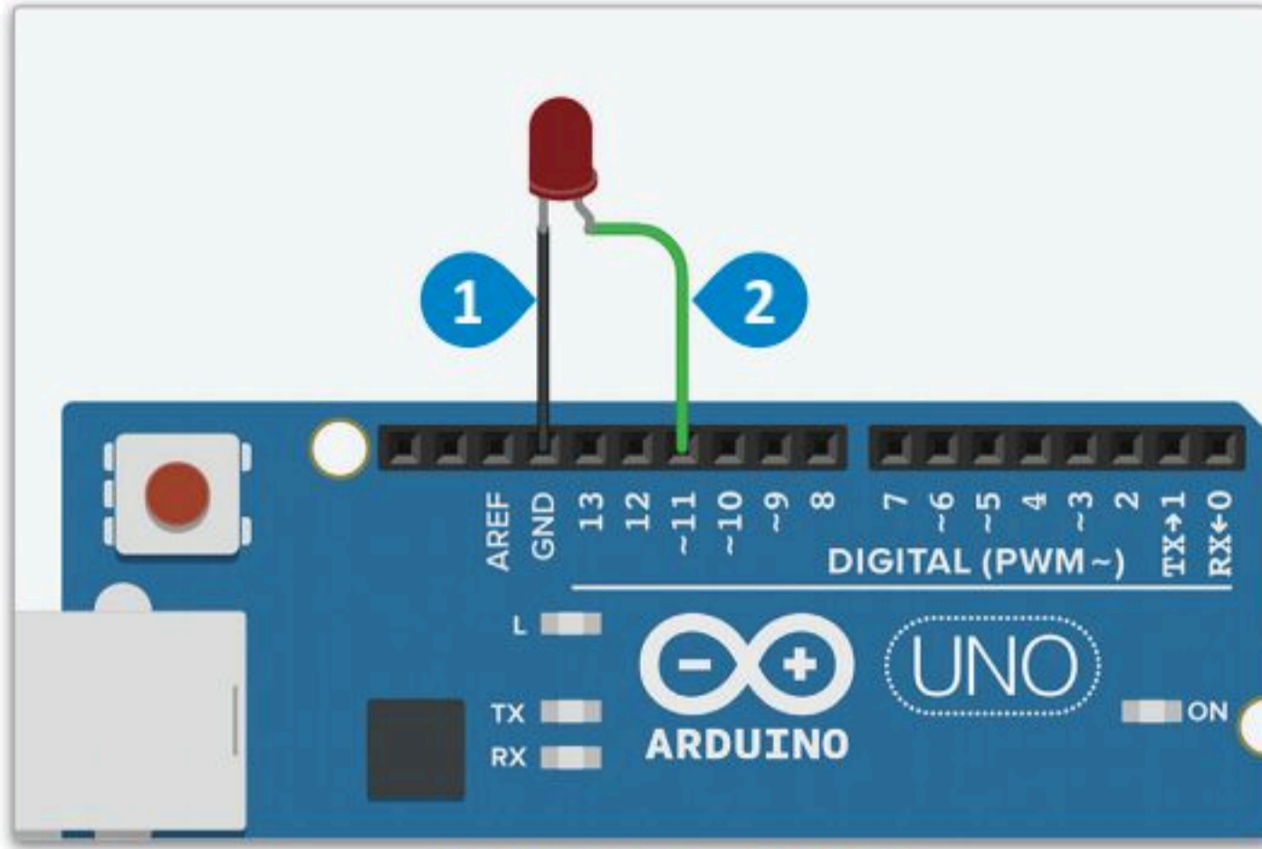
شكل 6.12: توصيل الـ LED المشع للضوء
