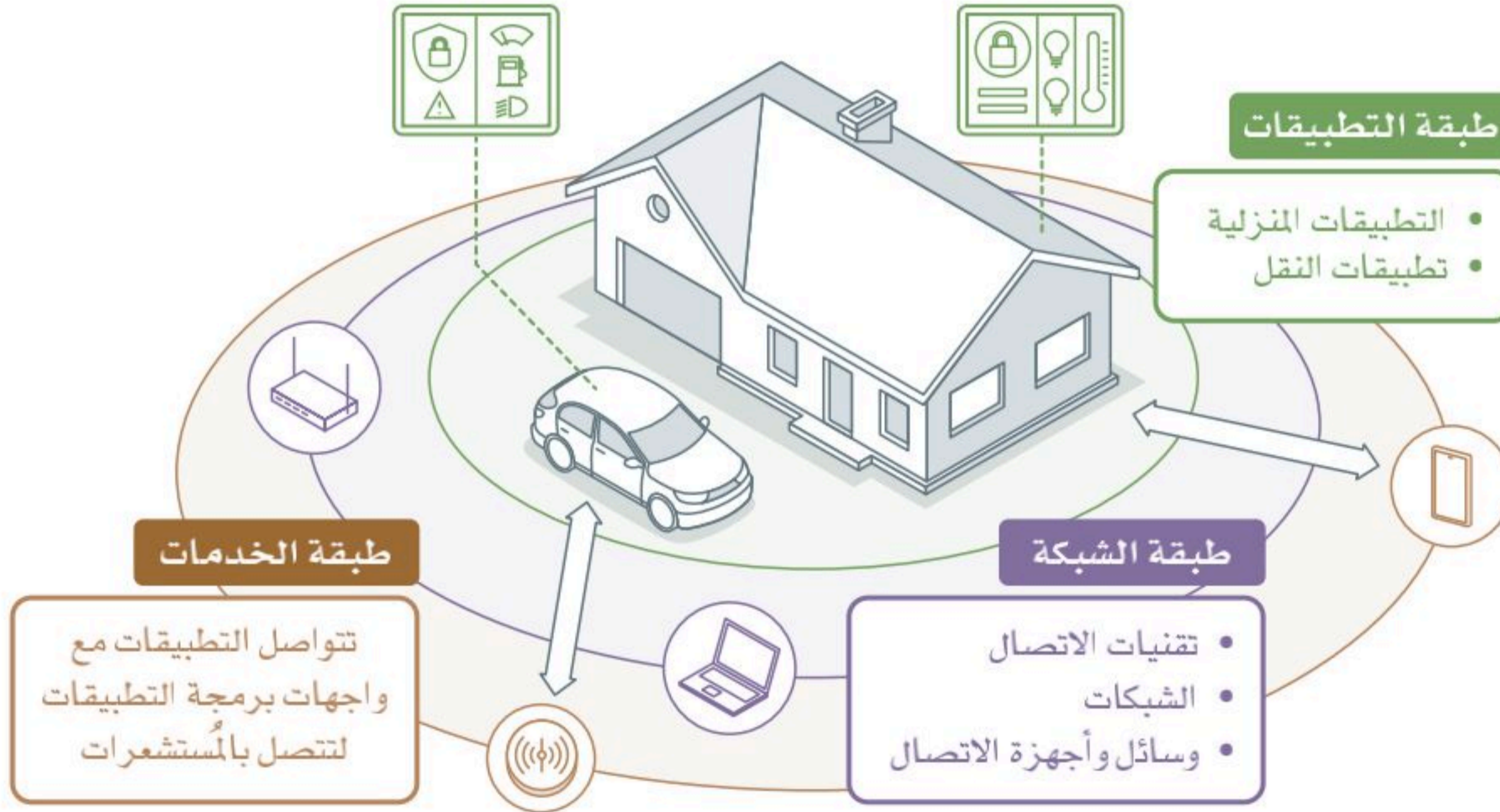
شكل 5.13: طبقات هيكلية oneM2M
