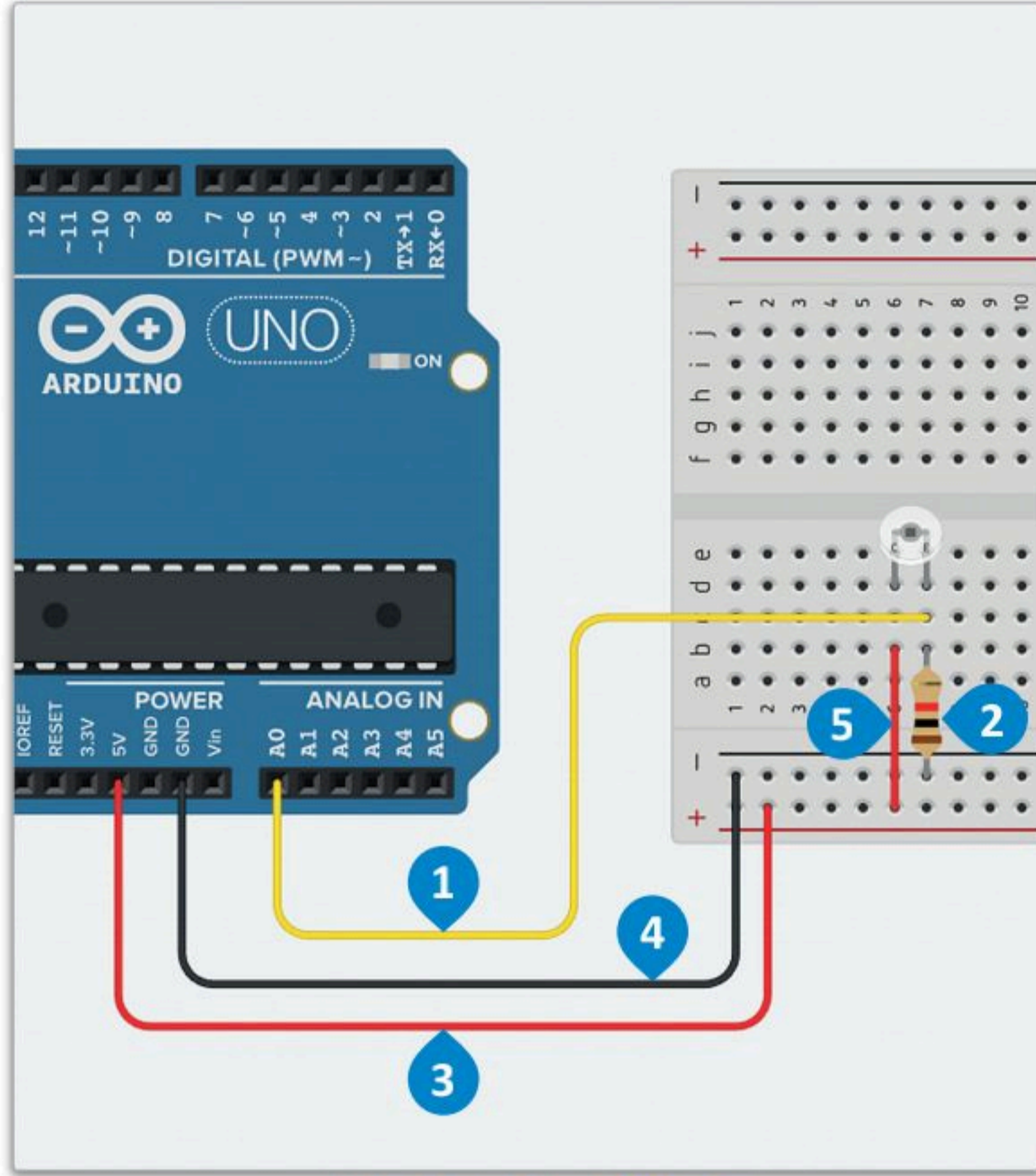
شكل 7.14: توصيل الترانزستور الضوئي
